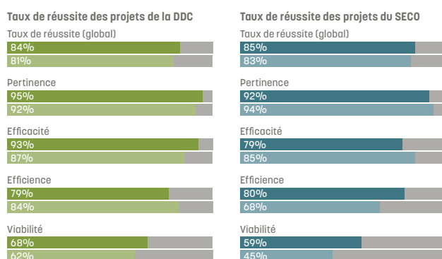
Schéma 2: taux de réussite, pertinence, efficacité, efficacité et viabilité des programmes et projets de la Direction du développement et de la coopération (DDC) et du Secrétariat d'État à l'économie (SECO), utilisant des méthodologies différentes. Une harmonisation des méthodologies est envisagée.
